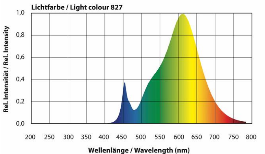
LED-Tropfenlampe G45
